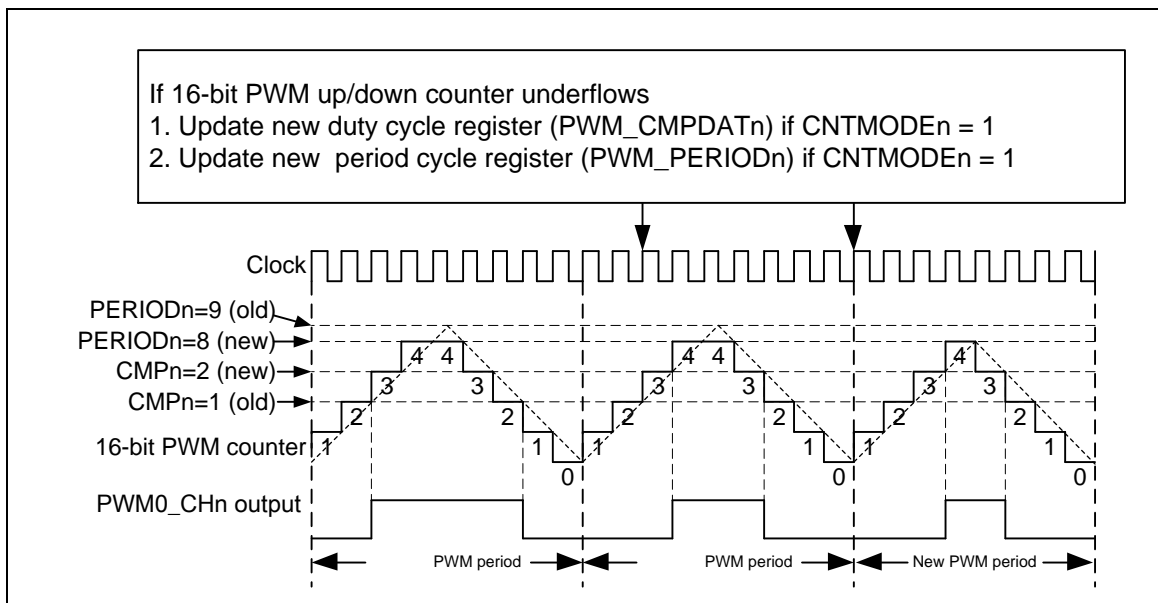
图 6.7-15 精确中心对齐模式
