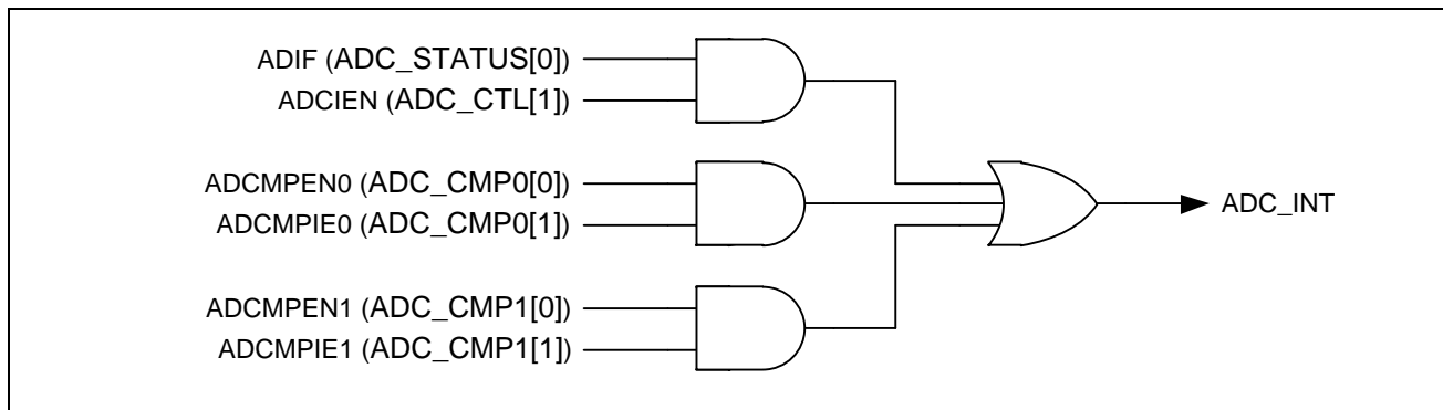
图 6.13-6 A/D控制器中断
