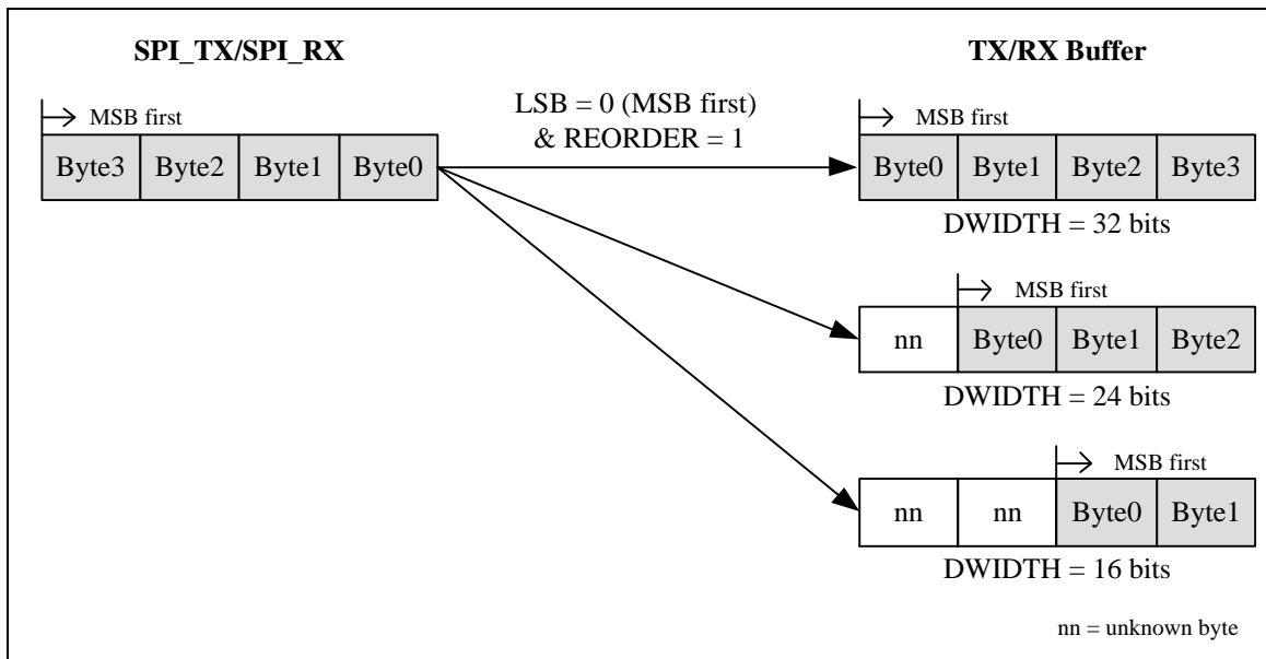
图 6.12-5 字节重排序
