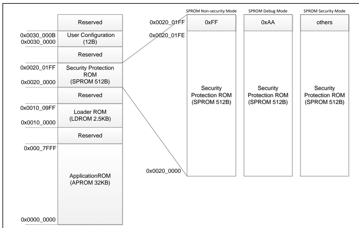
图 6.4-3 SPROM 安全锁模式
