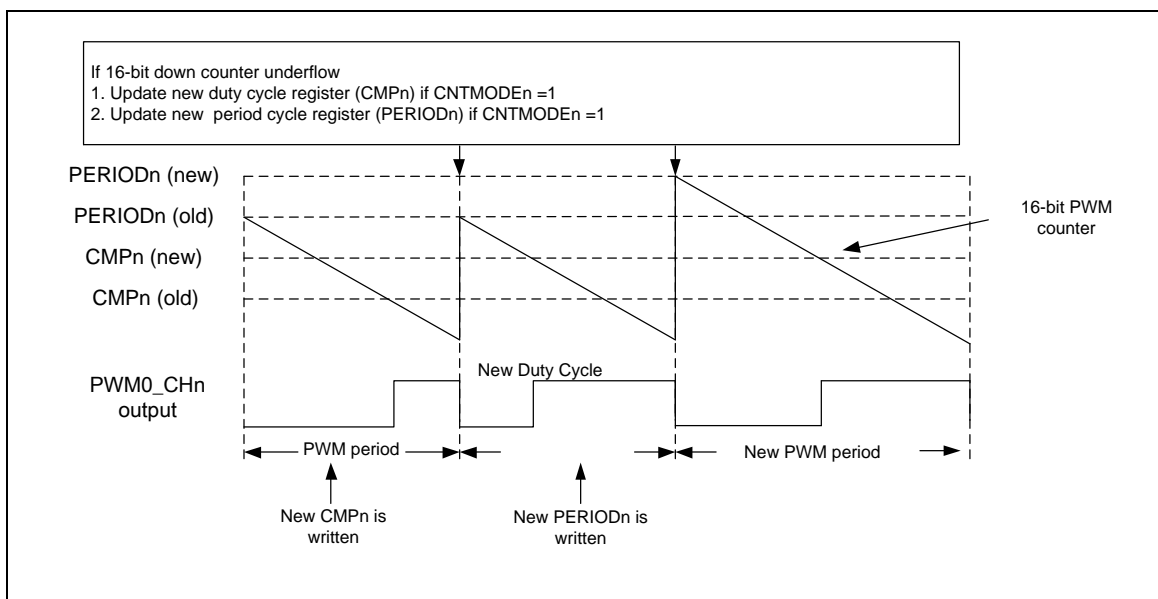
图 6.7-6 边沿对齐模式PWM
