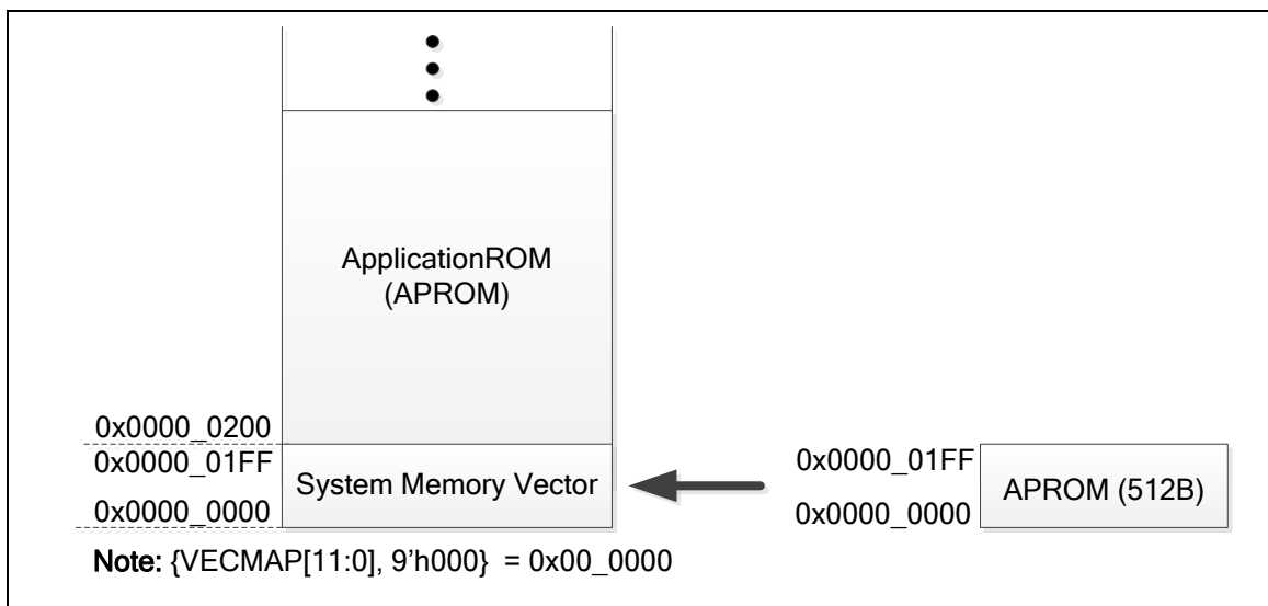
图 6.4-7 支持IAP的APROM模式
