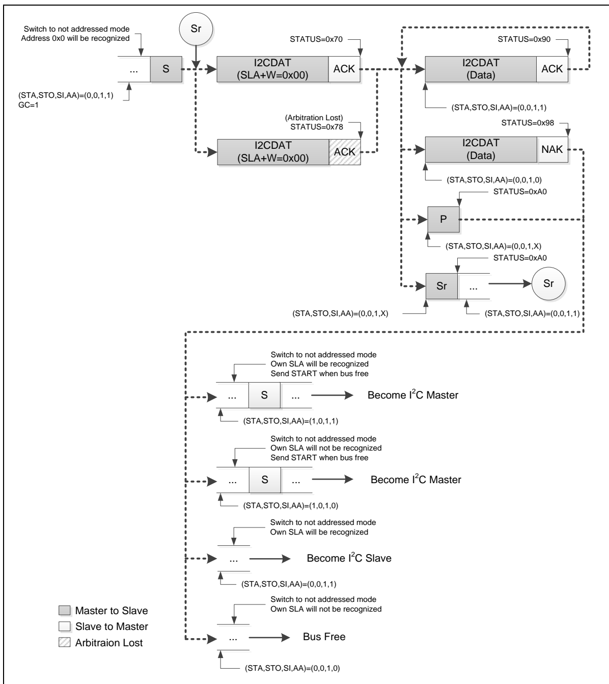
图 6.11-15 GC 模式
