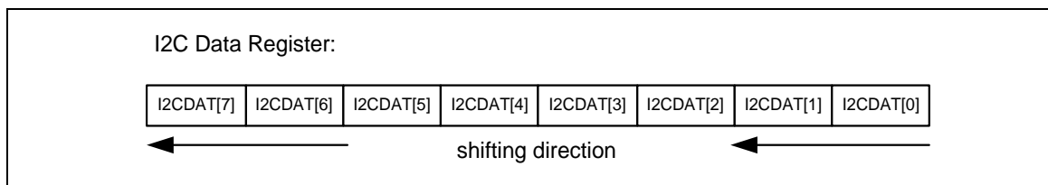
图 6.11-16 I2C 数据移动方向
