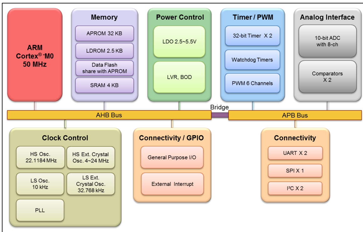
图 5.1-1 NuMicro® Mini58 系列方框图
