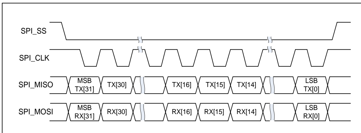
图 6.12-4 一次传输32-位
