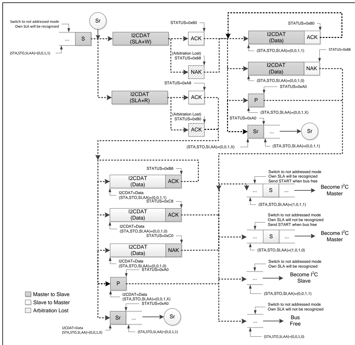
图 6.11-14 从机模式控制流程
