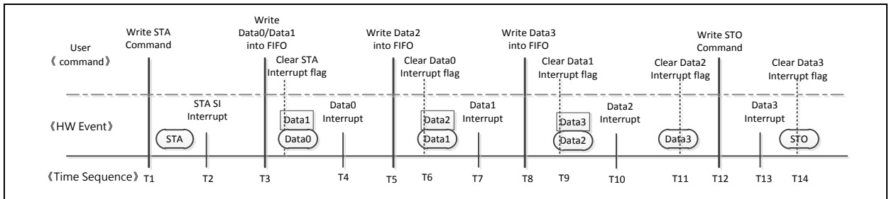
图 6.11-9 主机写时 二级缓存传输时序
