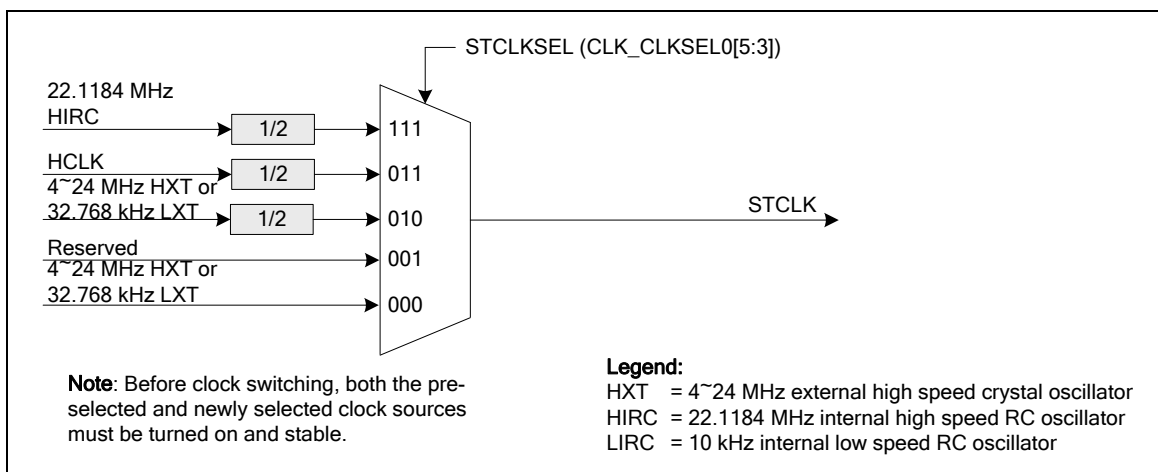
图 6.3-4 SysTick 时钟控制框图
