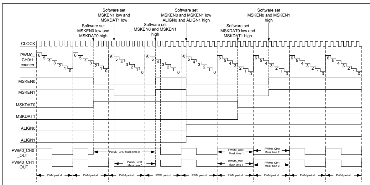
图 6.7-25 屏蔽和屏蔽对齐
