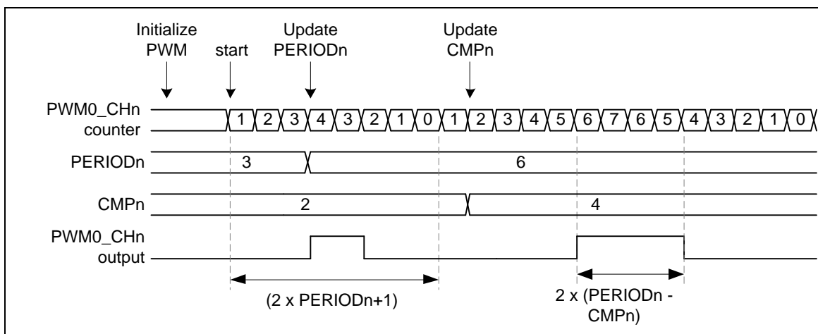
图 6.7-12 中心对齐模式时序图
