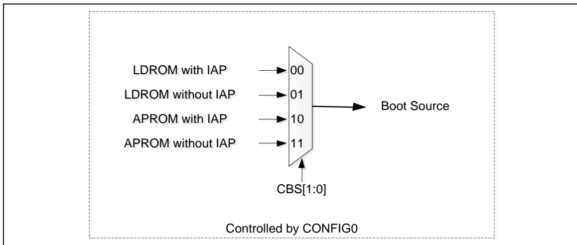
图 6.4-9 启动源选择
