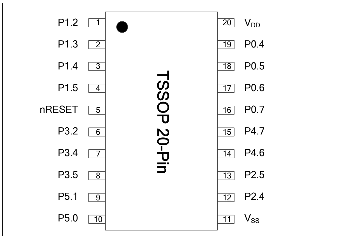
图 4.3-5 NuMicro® Mini58 系列 TSSOP 20-pin 管脚图
