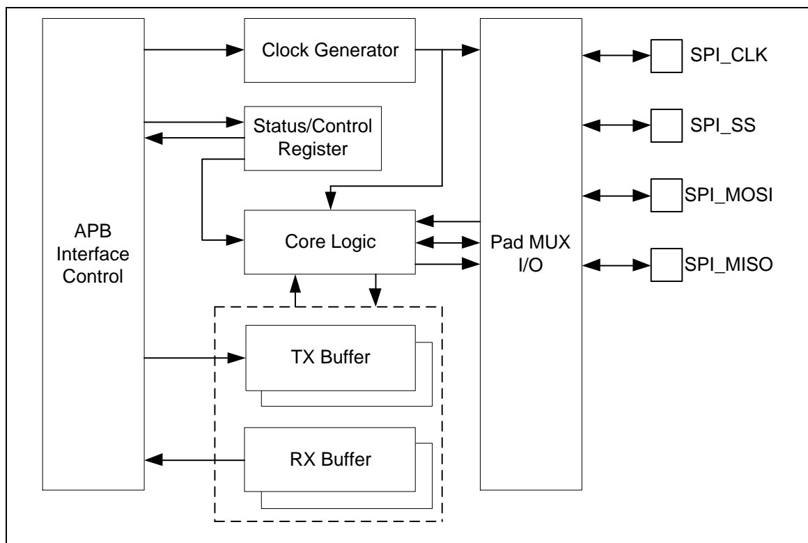
图 6.12-1 SPI 框图
