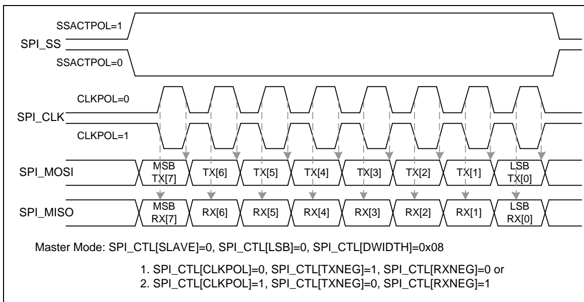
图 6.12-8 SPI 主机模式下的时序
