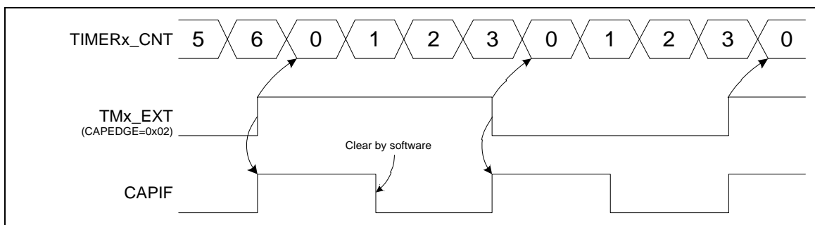
图 6.6-5 外部复位计数模式
