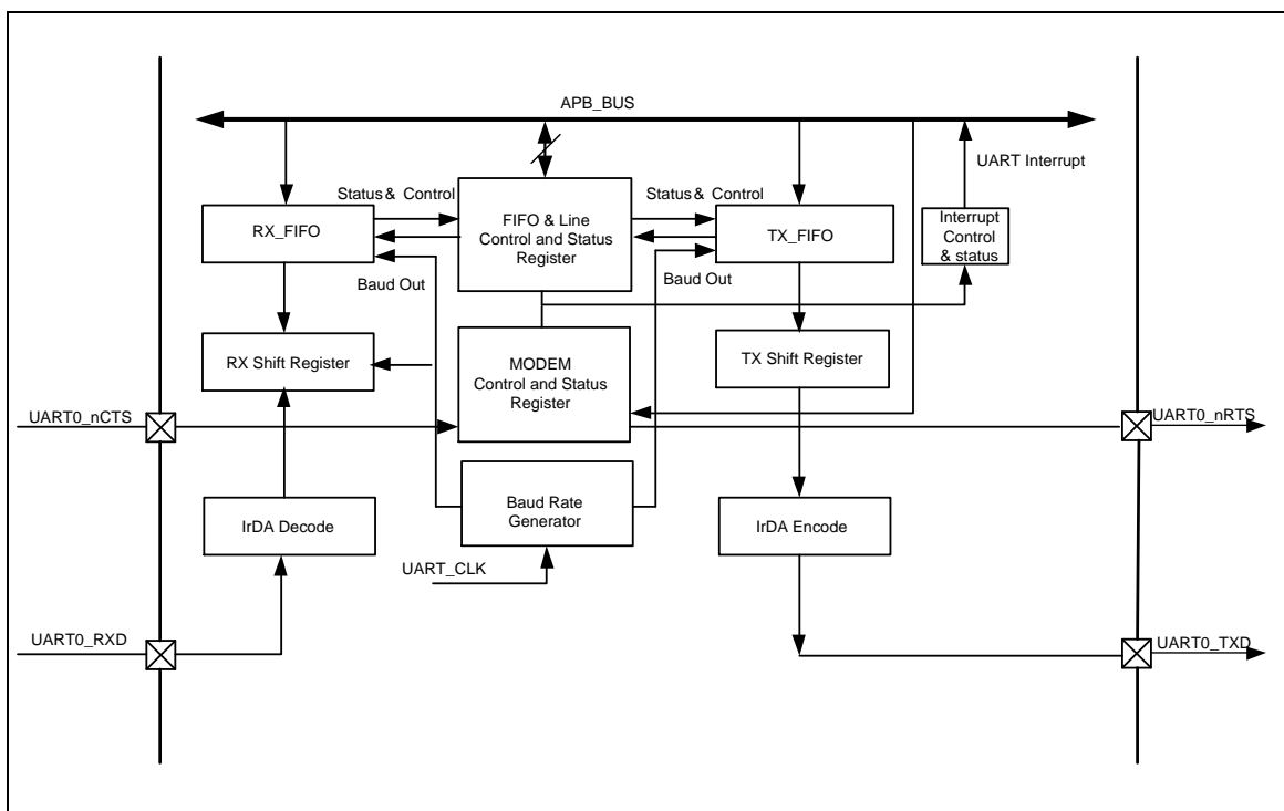
图 6.10-3 UART0 控制器框图
