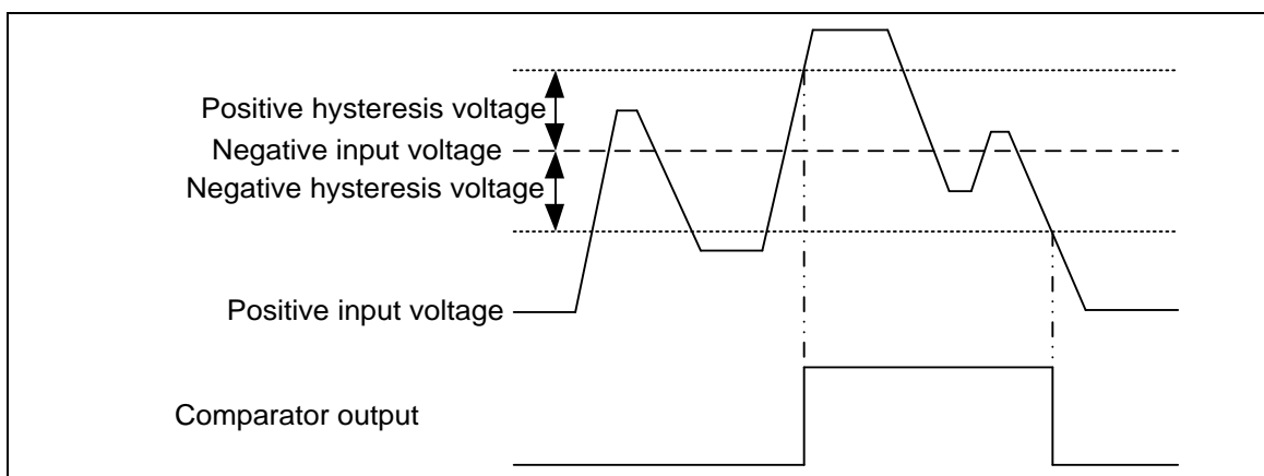
图 6.14-3 比较器的迟滞功能
