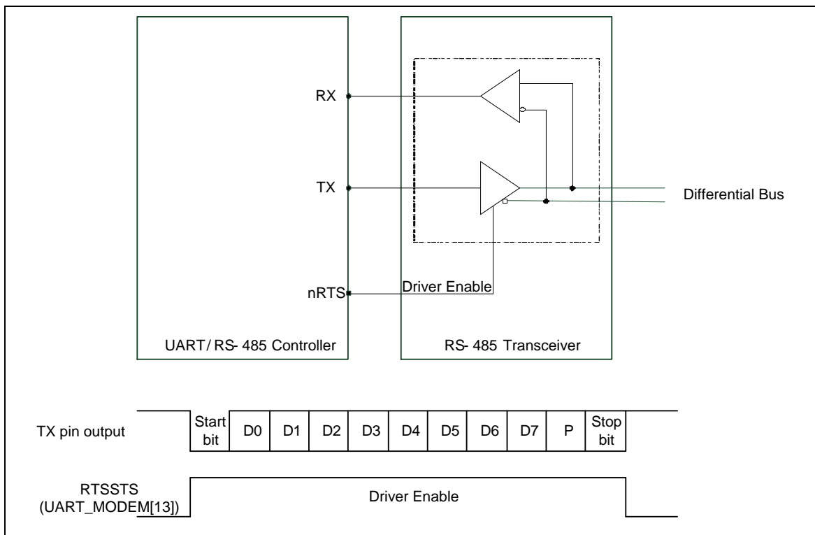
图 6.10-19 RS-485 帧结构
