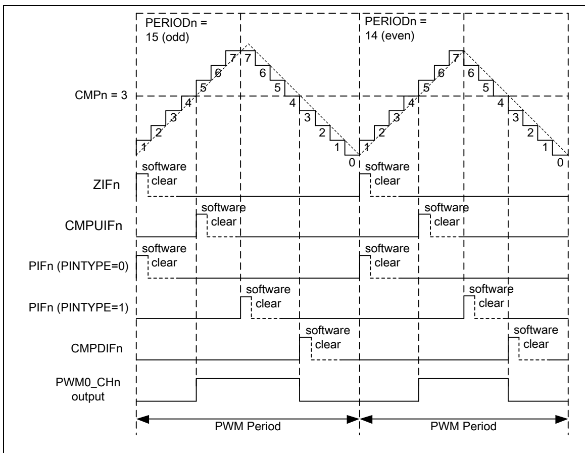
图 6.7-16 精确中心对齐波形图
