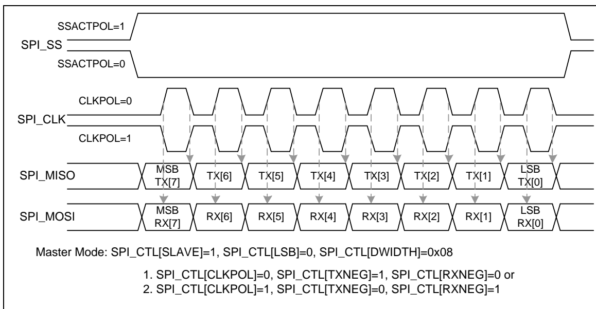
图 6.12-10 SPI从机模式下的时序
