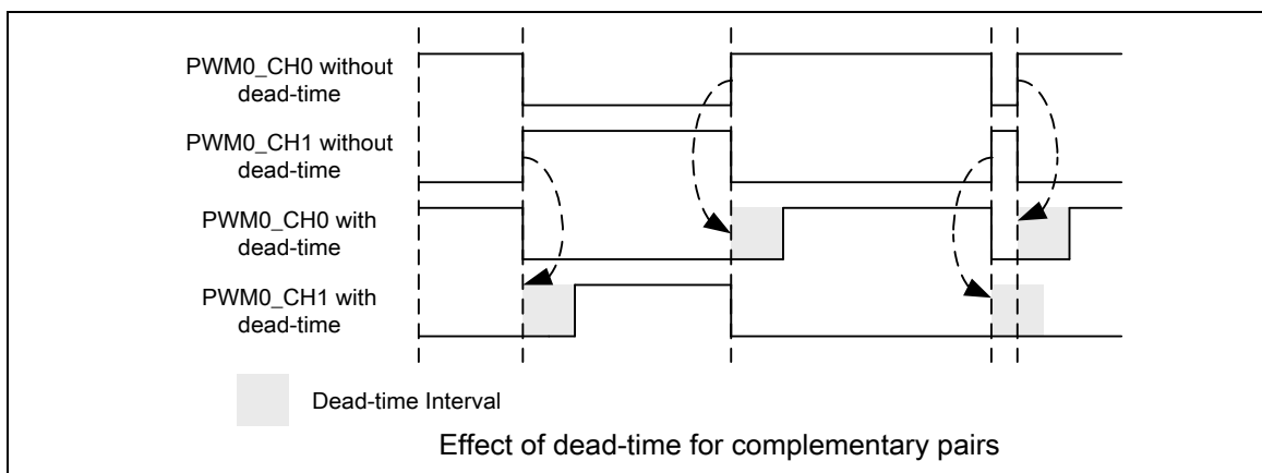
图 6.7-21 死区时间示意图
