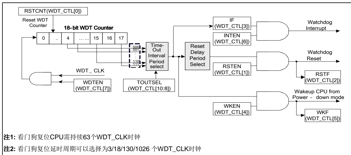
图 6.8-1 看门狗定时器模块图
