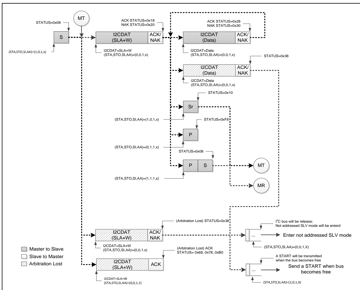
图 6.11-12 主机传送模式控制流程
