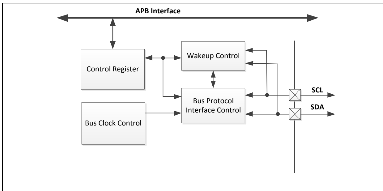
图 6.11-1 I 2 C 控制器框图
