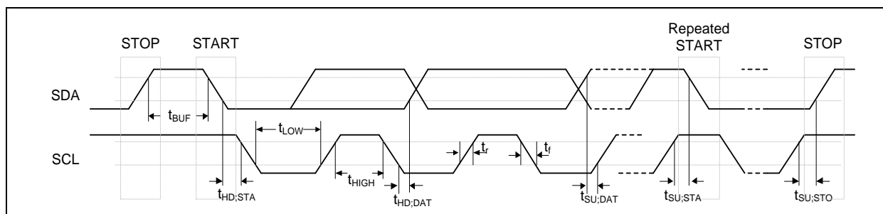
图 6.11-2 I 2 C 总线时序
