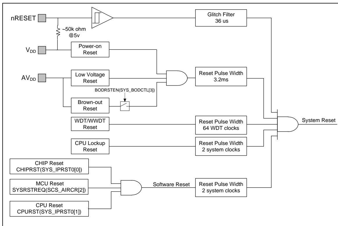
图 6.2-1 系统复位源
