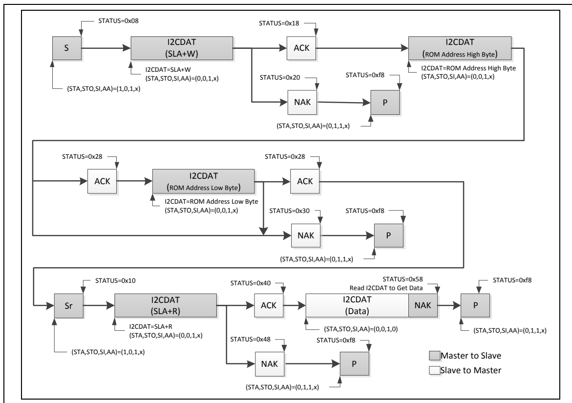
图 6.11-19 随机读协议
